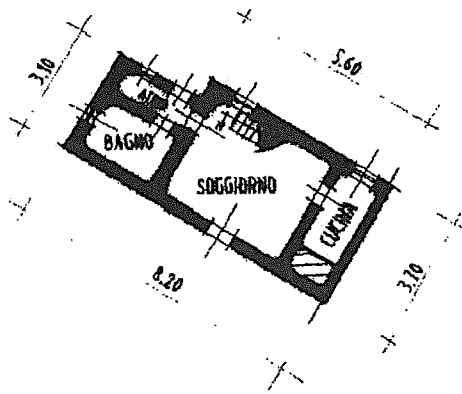
PIANTA PIANO TERRA h; 2.30
